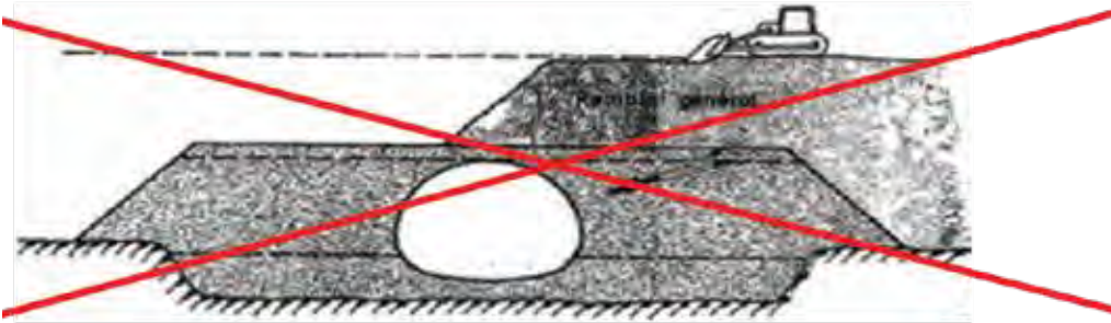
➤ Mise en œuvre dissymétrique du remblai général : A PROSCRIRE - Source : Publication SETRA / DRCR
