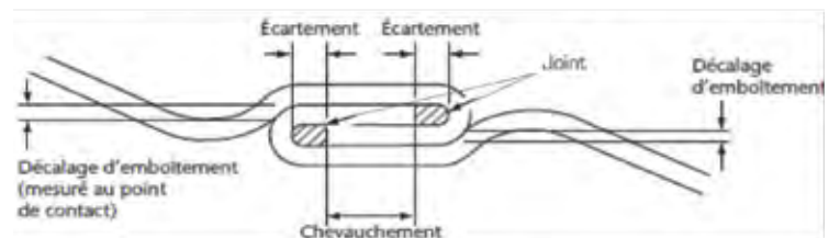
Coupe type d'un joint agrafé
