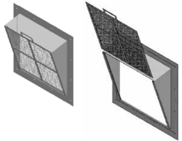
➔ Détail du FILTRAO® à positionner dans un regard carré Maille inox 1000 µm conformément à l'arrêté du 21 août 2008
